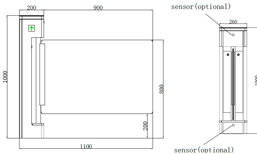
Abbildung 4 - Abmessungen des Produkts
